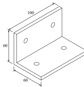
CODE 4276 CONNECTOR FOR GUIDE CLS-306 / JONCTION POUR GUIDAGE CLS-306 PRICE / PRIX 1,30 €/pc
