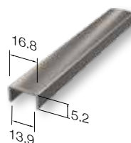
ΚΟΥΡΑΣΤΗ ΓΙΑ ΥΑΛΟΠΙΝΑΚΑ 6.6.2/6.6.4 HANDRAIL 6.6.2/6.6.4
