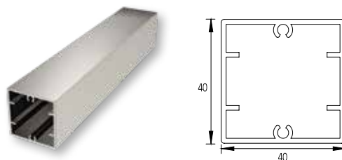
ΚΟΛΩΝΑ ΣΤΗΡΙΞΗΣ 40x40 SUPPORT COLUMN 40x40
