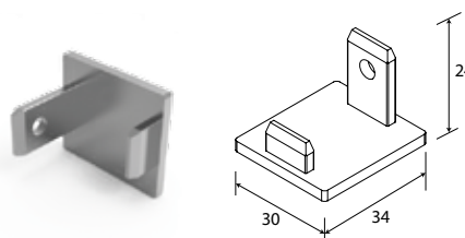
ΤΑΠΑ ΟΔΗΓΟΥ F50-319 END CAP FOR F50-319 GUIDE
