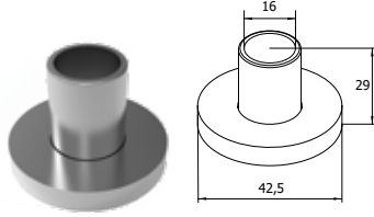
ΒΑΣΗ ΣΤΗΡΙΞΗΣ ΜΕ ΑΡΜΟΚΑΛΛΥΠΤΡΟ ΓΙΑ Ø16 CONNECTOR WITH COVER FOR PROFILE Ø16
