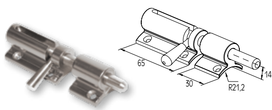
ΣΥΡΤΗΣ ΚΟΛΩΝΑΣ F50-100 BOLT FOR F50-100 COLUMN
