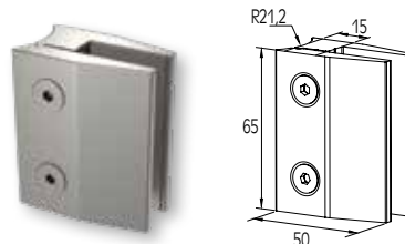
ΣΤΗΡΙΓΜΑ ΤΖΑΜΙΟΥ 8-10 mm GLASS SUPPORT 8-10mm
