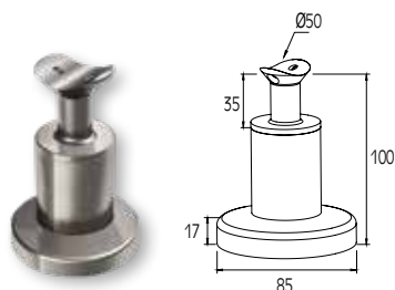
ΣΤΗΡΙΓΜΑ ΚΟΥΠΙΑΣΤΗΣ F50-200 SUPPORT FOR F50-200 HANDRAIL
