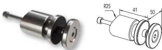
ΣΤΗΡΙΓΜΑ ΤΖΑΜΙΟΥ ΜΟΝΟ 8-10mm ΓΙΑ ΚΟΛΩΝΑ F50-101 SINGLE GLASS SUPPORT 8-10mm FOR F50-101 COLUMN
