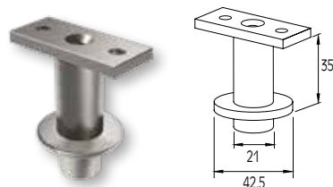
ΣΥΝΔΕΣΜΟΣ ΚΟΛΩΝΑΣ F50-100 ΜΕ ΚΟΥΠΙΑΣΤΗ F50-201 CONNECTOR FOR F50-100 COLUMN WITH F50-201 HANDRAIL
