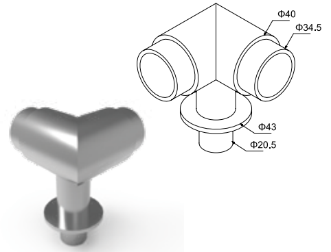
ΚΩΔ. / CODE 4262 ΣΥΝΔΕΣΜΟΣ 90° ΓΙΑ ΚΟΥΠΑΣΤΗ Ø40 CONNECTOR 90° FOR HANDRAIL Ø40 ΤΙΜΗ / PRICE 11,90 €/pc
