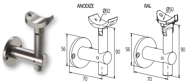
ΕΠΙΤΟΙΧΙΟ ΣΤΗΡΙΓΜΑ ΚΟΥΠΙΑΣΤΗΣ F50-200 WALL SUPPORT FOR F50-200 HANDRAIL WALL
