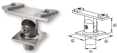
ΣΥΝΔΕΣΜΟΣ ΚΟΛΩΝΑΣ F50-102 ΜΕ ΚΟΥΠΑΣΤΗ F50-201 CONNECTOR FOR F50-102 COLUMN WITH F50-201 HANDRAIL
