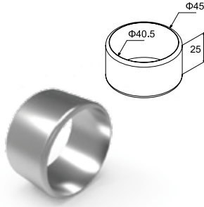
ΚΩΔ. / CODE 4260 ΣΥΝΔΕΣΜΟΣ ΚΟΥΠΑΣΤΗΣ Ø40 CONNECTOR FOR HANDRAIL Ø40 ΤΙΜΗ / PRICE 3,20 €/pc
