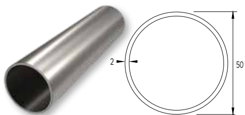
ΚΟΥΠΑΣΤΗ Ø50 HANDRAIL Ø50
