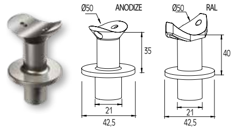
ΣΥΝΔΕΣΜΟΣ ΚΟΥΠΙΑΣΤΗΣ Ø50 ΜΕ ΚΟΛΩΝΑ Ø42 CONNECTOR FOR HANDRAIL Ø50 WITH COLUMN Ø42
