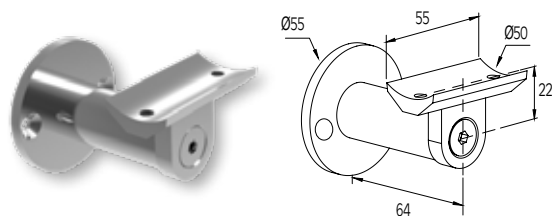
ΕΠΙΤΟΙΧΙΟ ΣΤΗΡΙΓΜΑ ΚΟΥΡΠΑΣΤΗΣ F50-200 WALL SUPPORT FOR F50-200 HANDRAIL
