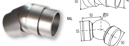
ΣΥΝΔΕΣΜΟΣ ΜΕΤΑΒΛΗΤΗΣ ΓΩΝΙΑΣ ΚΟΥΠΑΣΤΩΝ Ø50 ADJUSTABLE CORNER CONNECTOR FOR COLUMN Ø50
