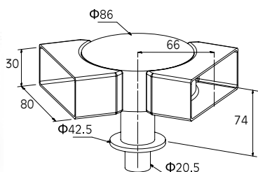
ΣΥΝΔΕΣΜΟΣ ΜΕΤΑΒΛΗΤΗΣ ΓΩΝΙΑΣ ΚΟΥΠΑΣΤΗΣ 80x30 ΜΕ ΚΟΛΩΝΑΣ F50-100 ADJUSTABLE CORNER CONNECTOR FOR HANDRAIL 80x30 WITH COLUMN F50-100
