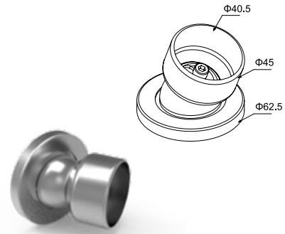
ΚΩΔ. / CODE 4521 ΑΡΜΟΚΑΛΥΠΤΡΟ ΚΟΥΠΑΣΤΗΣ Ø40 (ΜΕ ΚΑΠΑΚΙ) WALL COVER FOR HANDRAIL Ø40 WITH CAP ΤΙΜΗ / PRICE 10,10 €/pc
