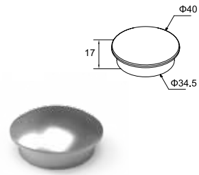
ΚΩΔ. / CODE 4479 ΤΑΠΑ ΚΟΥΠΑΣΤΗΣ Ø40 END CAP FOR HANDRAIL Ø40 ΤΙΜΗ / PRICE 1,30 €/pc
