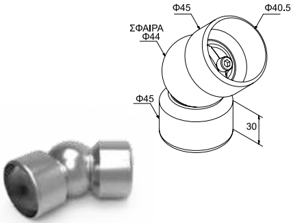
ΚΩΔ. / CODE 4367 ΣΥΝΔΕΣΜΟΣ ΜΕΤΑΒΛΗΤΗΣ ΓΩΝΙΑΣ ΚΟΥΠΑΣΤΗΣ Ø40 ADJUSTABLE CORNER CONNECTOR FOR HANDRAIL Ø40 ΤΙΜΗ / PRICE 8,30 €/pc
