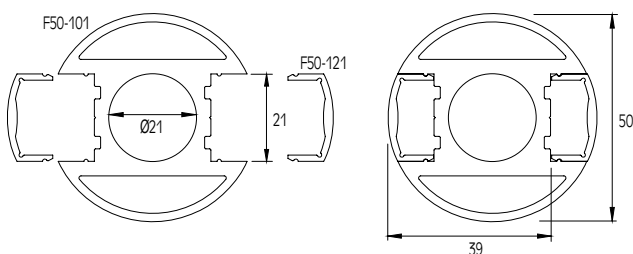
ΚΑΠΑΚΙ ΚΟΛΩΝΑΣ F50-101 COVER FOR F50-101 COLUMN
