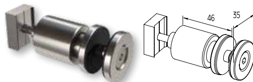
ΣΤΗΡΙΓΜΑ ΤΖΑΜΙΟΥ ΜΟΝΟ 8-10mm ΓΙΑ ΚΟΛΩΝΑ BLADE SINGLE GLASS SUPPORT 8-10mm FOR BLADE COLUMN
