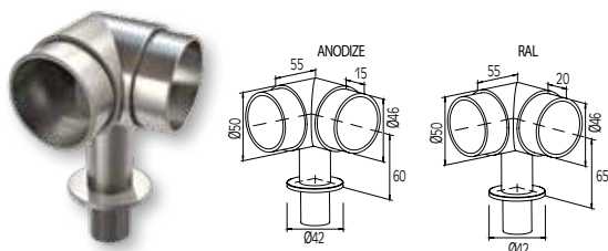
ΣΥΝΔΕΣΜΟΣ 90° ΓΙΑ ΚΟΥΠΙΑΣΤΗ Ø50 CONNECTOR 90° FOR HANDRAIL Ø50
