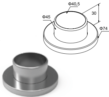
ΑΡΜΟΚΑΛΥΠΤΡΟ ΚΟΥΠΑΣΤΗΣ Ø40 WALL COVER FOR HANDRAIL Ø40 ΚΩΔ. / CODE 4520Z ΤΙΜΗ / PRICE 5,45 €/pc
