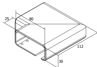
ΣΥΝΔΕΣΜΟΣ 90° ΚΟΥΠΑΣΤΩΝ 80X30 CONNECTOR 90° 80X30 HANDRAIL
