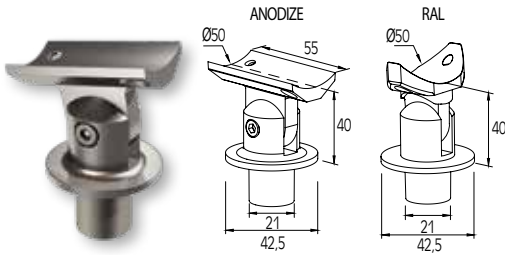
ΣΥΝΔΕΣΜΟΣ ΚΟΥΠΙΑΣΤΗΣ Ø50 ΜΕ ΚΟΛΩΝΑ Ø42 (ΣΚΑΛΑ) CONNECTOR FOR HANDRAIL Ø50 WITH COLUMN Ø42 (STAIRS)
