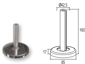
ΠΕΛΜΑ ΣΤΗΡΙΞΗΣ ΓΙΑ ΚΟΛΩΝΑ Ø42 SUPPORT FOOT FOR Ø42 COLUMN
