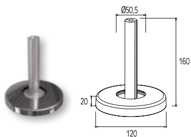
ΠΕΛΜΑ ΣΤΗΡΙΞΗΣ ΓΙΑ ΚΟΛΩΝΑ Ø50 SUPPORT FOOT FOR Ø50 COLUMN
