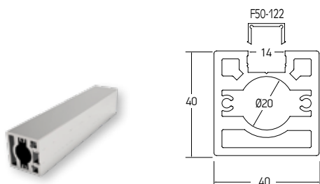
ΚΟΛΩΝΑ ΣΤΗΡΙΞΗΣ 40x40 SUPPORT COLUMN 40x40
