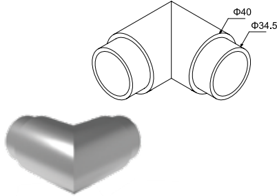
ΚΩΔ. / CODE 4277 ΣΥΝΔΕΣΜΟΣ 90° ΓΙΑ ΚΟΥΠΑΣΤΗ Ø40 CONNECTOR 90° FOR HANDRAIL Ø40 ΤΙΜΗ / PRICE 6,95 €/pc
