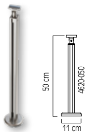
ΕΤΟΙΜΗ ΚΟΛΩΝΑ 50 cm ΓΙΑ ΠΡΟΦΙΛ Ø16 READY MADE COLUMN FOR Ø16 PROFILE HEIGHT 50 cm
