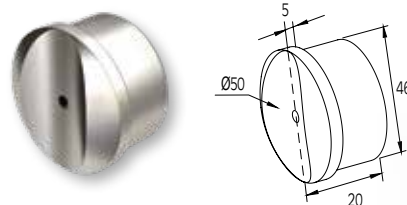
ΣΥΝΔΕΣΜΟΣ ΚΟΥΠΑΣΤΗΣ - ΚΟΥΠΑΣΤΗΣ F50-200 CONNECTOR FOR HANDRAIL WITH HANDRAIL F50-200
