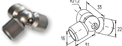
ΣΥΝΔΕΣΜΟΣ ΜΕΤΑΒΛΗΤΗΣ ΓΩΝΙΑΣ ΠΡΟΦΙΛ Ø16 ΜΕ ΚΟΛΩΝΑ F50-100 ADJUSTABLE CORNER CONNECTOR FOR PROFILE Ø16 WITH F50-100 COLUMN
