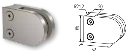
ΣΤΗΡΙΓΜΑ ΤΖΑΜΙΟΥ 6-8mm INOX GLASS SUPPORT 6-8mm
