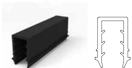
ΛΑΣΤΙΧΟ ΣΦΗΝΑ ΟΔΗΓΟΥ ΤΥΠΟΥ U ΓΙΑ ΤΖΑΜΙ 10.76mm "U" SHAPE GASKET FOR 10.76mm GLASS
