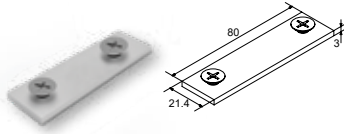
ΕΥΘΕΙΑ ΓΩΝΙΑ ΣΥΝΔΕΣΗΣ ΟΔΗΓΟΥ F50-319 LINEAR CONNECTOR FOR F50-319 GUIDE
