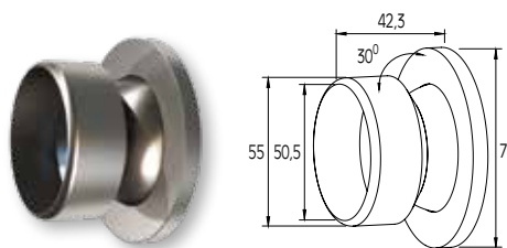
ΑΡΜΟΚΑΛΥΠΤΡΟ ΚΟΥΠΙΑΣΤΗΣ Ø50 (ΜΕ ΚΑΠΑΚΙ) WALL COVER FOR HANDRAIL Ø50 WITH CAP
