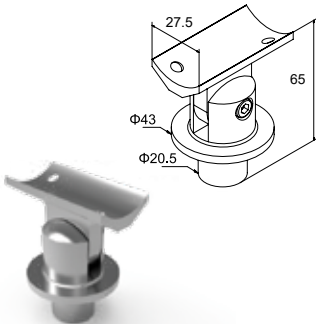
ΚΩΔ. / CODE 4369 ΣΤΗΡΙΓΜΑ ΜΕΤΑΒΛΗΤΗΣ ΓΩΝΙΑΣ ΚΟΥΠΑΣΤΗΣ Ø40 ΜΕ ΚΟΛΩΝΑ Ø42 ADJUSTABLE CORNER SUPPORT FOR HANDRAIL Ø40 WITH COLUMN Ø42 ΤΙΜΗ / PRICE 6,40 €/pc
