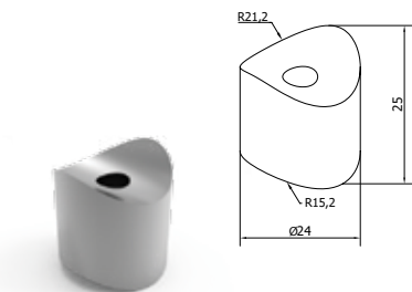
ΣΥΝΔΕΣΜΟΣ F50-307/327 ΜΕ ΚΟΛΩΝΑ F50-103/123 CONNECTOR FOR F50/307-327 WITH F50-103/123 COLUMN
