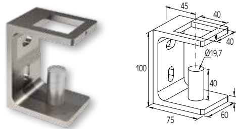
ΕΞΩΤΕΡΙΚΟ ΣΤΗΡΙΓΜΑ ΚΟΛΩΝΑΣ F50-102 EXTERNAL SUPPORT FOR F50-102 COLUMN
