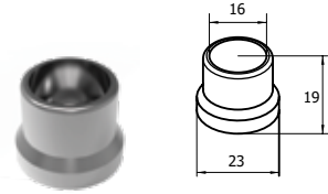
ΒΑΣΗ ΣΤΗΡΙΞΗΣ ΓΙΑ Ø16 CONNECTOR FOR PROFILE Ø16
