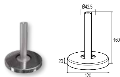
ΠΕΛΜΑ ΣΤΗΡΙΞΗΣ ΓΙΑ ΚΟΛΩΝΑ Ø42 SUPPORT FOOT FOR Ø42 COLUMN
