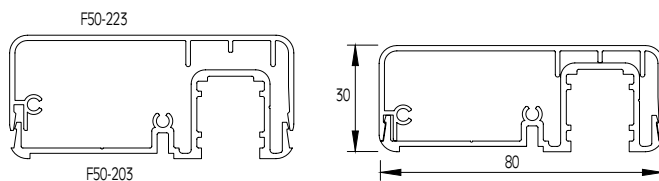
ΚΑΠΑΚΙ ΔΙΑΙΡΟΥΜΕΝΗΣ ΚΟΥΠΑΣΤΗΣ F50-203 COVER FOR DIVIDABLE HANDRAIL F50-203
