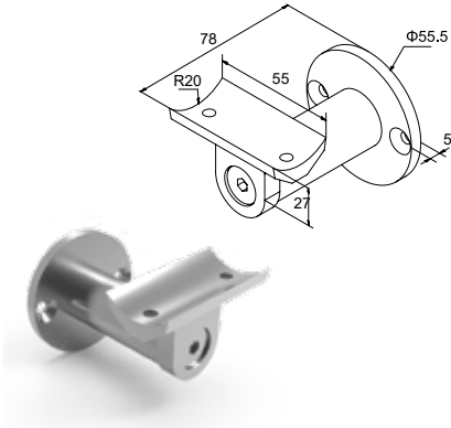
ΚΩΔ. / CODE 4135 ΕΠΙΤΟΙΧΙΟ ΣΤΗΡΙΓΜΑ ΚΟΥΠΑΣΤΗΣ Ø40 WALL SUPPORT FOR Ø40 HANDRAIL ΤΙΜΗ / PRICE 6,05 €/pc
