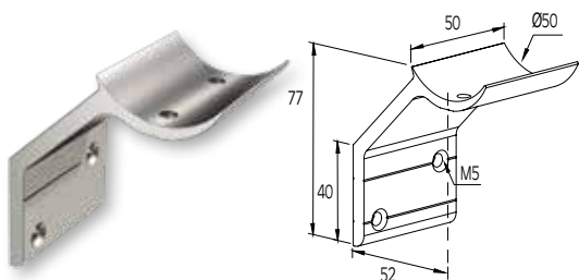
ΕΠΙΤΟΙΧΙΟ ΣΤΑΘΕΡΟ ΣΤΗΡΙΓΜΑ ΚΟΥΡΠΑΣΤΗΣ F50-200 FIXED WALL SUPPORT FOR F50-200 HANDRAIL
