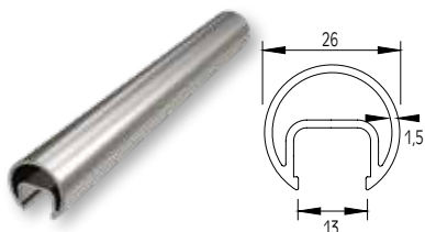
ΟΔΗΓΟΣ ΓΙΑ ΤΖΑΜΙ GUIDE FOR GLASS
