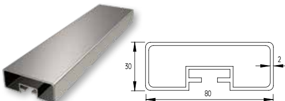
ΚΟΥΠΑΣΤΗ 30x80 HANDRAIL 30x80
