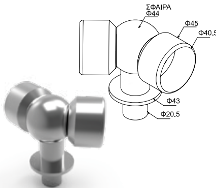
ΚΩΔ. / CODE 4370 ΣΥΝΔΕΣΜΟΣ ΜΕΤΑΒΛΗΤΗΣ ΓΩΝΙΑΣ ΚΟΥΠΑΣΤΗΣ Ø40 ΜΕ ΚΟΛΩΝΑ Ø42 ADJUSTABLE CORNER CONNECTOR FOR HANDRAIL Ø40 WITH COLUMN Ø42 ΤΙΜΗ / PRICE 19,20 €/pc
