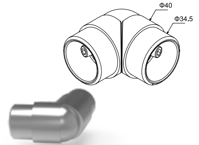
ΚΩΔ. / CODE 4371 ΣΥΝΔΕΣΜΟΣ ΜΕΤΑΒΛΗΤΗΣ ΓΩΝΙΑΣ ΚΟΥΠΑΣΤΗΣ Ø40 ADJUSTABLE CORNER CONNECTOR FOR HANDRAIL Ø40 ΤΙΜΗ / PRICE 9,55 €/pc
