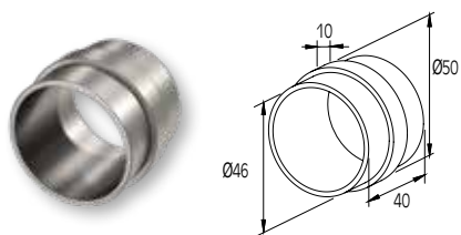
ΕΣΩΤΕΡΙΚΟΣ ΣΥΝΔΕΣΜΟΣ ΚΟΥΡΠΑΣΤΩΝ Ø50 CONNECTOR FOR HANDRAIL Ø50 (INTERNAL)
