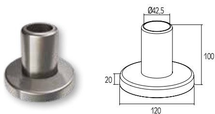
ΕΞΩΤΕΡΙΚΟ ΠΕΛΜΑ ΣΤΗΡΙΞΗΣ ΓΙΑ ΚΟΛΩΝΑ Ø42 EXTERNAL SUPPORT FOOT FOR Ø42 COLUMN
