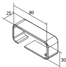
ΣΥΝΔΕΣΜΟΣ ΚΟΥΠΑΣΤΩΝ 80X30 ΕΥΘΕΙΑ CONNECT.FOR 80X30 HANDR. (STRAIGHT)
