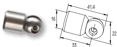
ΣΥΝΔΕΣΜΟΣ ΡΟΖΕΤΑΣ ΤΖΑΜΙΟΥ ΜΕ ΠΡΟΦΙΛ Ø16 CONNECTOR FOR GLASS ROSSETE WITH PROFILE Ø16
