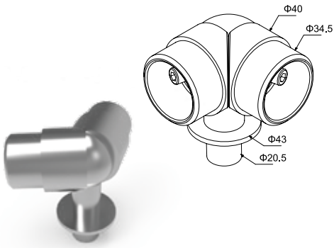
ΚΩΔ. / CODE 4372 ΣΥΝΔΕΣΜΟΣ ΜΕΤΑΒΛΗΤΗΣ ΓΩΝΙΑΣ ΚΟΥΠΑΣΤΗΣ Ø40 ΜΕ ΚΟΛΩΝΑ Ø42 ADJUSTABLE CORNER CONNECTOR FOR HANDRAIL Ø40 WITH COLUMN Ø42 ΤΙΜΗ / PRICE 15,10 €/pc
