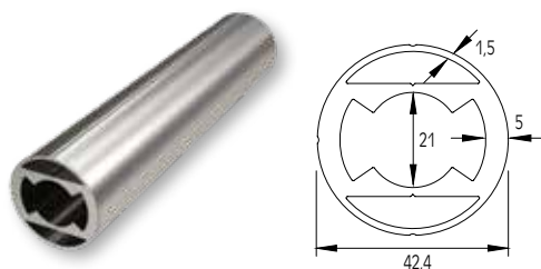
ΚΟΛΩΝΑ ΣΤΗΡΙΞΗΣ Ø42 ΕΝΙΣΧΥΜΕΝΗ SUPPORT COLUMN Ø42 (HEAVY-DUTY)
