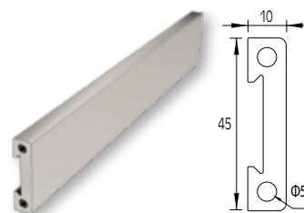
ΠΡΟΦΙΛ ΚΟΛΩΝΑΣ BLADE BLADE COLUMN
