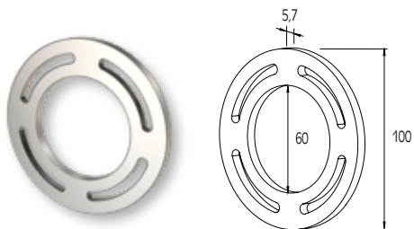
ΠΟΖΕΤΑ ΤΖΑΜΙΟΥ Ø100 GLASS ROSETTE Ø100
