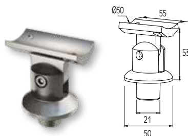
ΣΤΗΡΙΓΜΑ ΚΟΥΠΑΣΤΗΣ F50-200 ΜΕ ΚΟΛΩΝΑ F50-101 SUPPORT FOR HANDRAIL F50-200 WITH COLUMN F50-101
