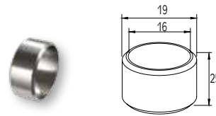
CONNECTOR FOR PROFILE Ø16 (STRAIGHT) JONCTION DE PROFIL Ø16 (DROIT)
