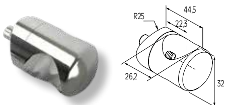
CONNECTOR OVAL FOR F50-101 COLUMN WITH PROFILE Ø26 JONCTION OVALE DE MAIN COURANTE F50-101 AVEC PROFIL Ø26
