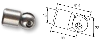
CONNECTOR FOR GLASS ROSSETTE WITH PROFILE Ø16 JONCTION DE ROSACE DE VERRE AVEC PROFIL Ø16
