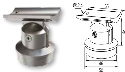
CONNECTOR FOR F50-100 COLUMN WITH F50-200 HANDRAIL JONCTION DE MAIN COURANTE F50-100 AVEC POTEAU F50-200
