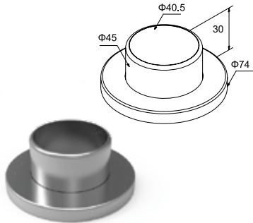
WALL COVER FOR HANDRAIL Ø40 CACHE DU MUR DE MAIN COURANTE Ø40 CODE 4520Z PRICE / PRIX 5,45 €/pc
