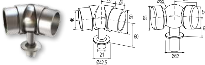
ADJUSTABLE CORNER CONNECTOR FOR HANDRAIL Ø50 WITH COLUMN Ø42 JONCTION ANGULAIRE DE MAIN COURANTE Ø50 AVEC POTEAU Ø42
