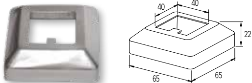
WALL COVER FOR F50-102 COLUMN CACHE DU MUR DE POTEAU F50-102
