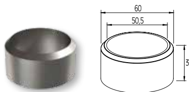
WALL COVER FOR F50-101 COLUMN CACHE DU MUR DE POTEAU F50-101
