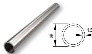
PROFILE Ø16x1.3 PROFIL Ø16x1.3
