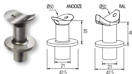
CONNECTOR FOR HANDRAIL Ø50 WITH COLUMN Ø42 JONCTION DE MAIN COURANTE Ø50 AVEC POTEAU Ø42
