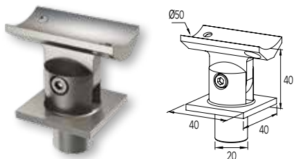
SUPPORT FOR F50-200 HANDRAIL WITH F50-102 COLUMN (STAIRS) FIXATION DE MAIN COURANTE F50-200 AVEC POTEAU F50-102 (ESCALIER)
