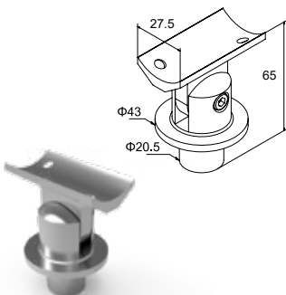
CODE 4369 ADJUSTABLE CORNER SUPPORT FOR HANDRAIL Ø40 WITH COLUMN Ø42 FIXATION ANGULAIRE DE MAIN COURANTE Ø40 AVEC POTEAU Ø42 PRICE / PRIX 6,40 €/pc
