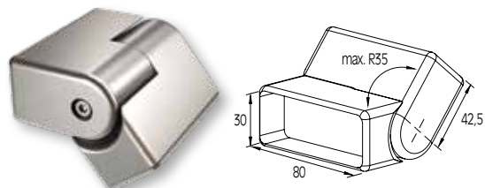
ADJUSTABLE CORNER CONNECTOR FOR 80x30 HANDRAIL (STAIRS) JONCTION ANGULAIRE DE POTEAU 80x30 (ESCALIER)
