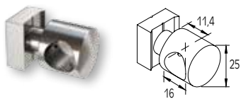
CONNECTOR FOR PROFILE Ø16 WITH BLADE COLUMN JONCTION DE PROFIL Ø16 AVEC POTEAU BLADE
