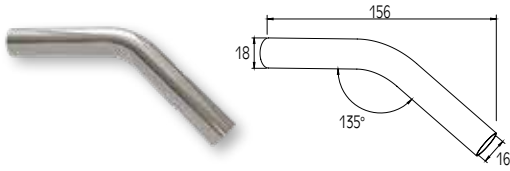
CONNECTOR 135° FOR PROFILE Ø16 JONCTION 135° DE PROFIL Ø16
