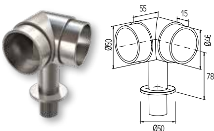
CONNECTOR 90° FOR HANDRAIL Ø50 JONCTION 90° DE MAIN COURANTE Ø50
