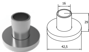
CONNECTOR WITH COVER FOR PROFILE Ø16 CONNECTEUR AVEC CAPUCHON POUR PROFIL Ø16
