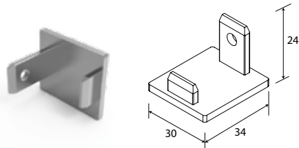
END CAP FOR F50-319 GUIDE EMBOUT DE GUIDAGE F50-319
