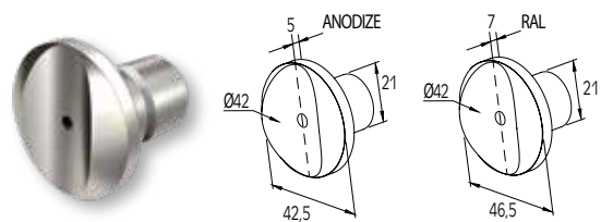
CONNECTOR FOR COLUMN WITH COLUMN F50-100 JONCTION DE POTEAU AVEC POTEAU F50-100
