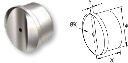
CONNECTOR FOR HANDRAIL WITH HANDRAIL F50-200 JONCTION DE MAIN COURANTE AVEC MAIN COURANTE F50-200
