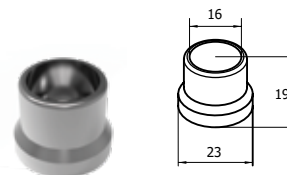
CONNECTOR FOR PROFILE Ø16 CONNECTEUR POUR PROFIL Ø16
