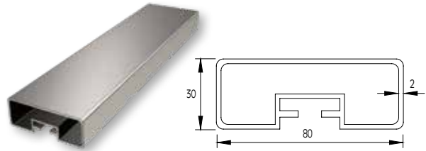
HANDRAIL 30x80 MAIN COURANTE 30x80
