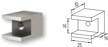
CONNECTOR FOR F50-102/106 COLUMN WITH PROFILE F50-302 JONCTION DE POTEAU F50-102/106 AVEC PROFIL F50-302
