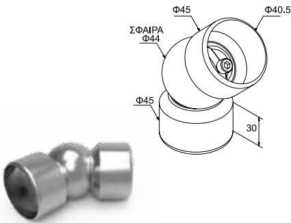
CODE 4367 ADJUSTABLE CORNER CONNECTOR FOR HANDRAIL Ø40 JONCTION ANGULAIRE DE MAIN COURANTE Ø40 PRICE / PRIX 8,30 €/pc
