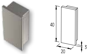
END CAP FOR PROFILE 59-009 (40x20) EMBOUT DE PROFIL 59-009 (40x20)
