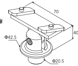
SUPPORT FOR F50-201 HANDRAIL WITH F50-100 COLUMN (STAIRS) FIXATION DE MAIN COURANTE F50-201 AVEC POTEAU F50-100(ESCALIER)
