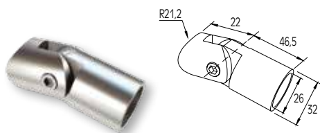
CONNECTOR FOR F50-100 COLUMN WITH PROFILE Ø26 JONCTION DE POTEAU F50-100 AVEC PROFIL Ø26
