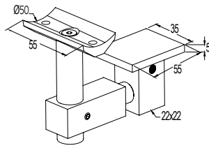
SUPPORT FOR HANDRAIL Ø50 WITH BLADE COLUMN FIXATION DE MAIN COURANTE Ø50 AVEC POTEAU BLADE
