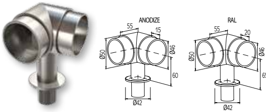
CONNECTOR 90° FOR HANDRAIL Ø50 JONCTION 90° DE MAIN COURANTE Ø50
