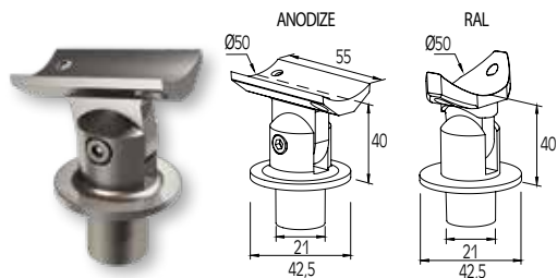
CONNECTOR FOR HANDRAIL Ø50 WITH COLUMN Ø42 (STAIRS) JONCTION DE MAIN COURANTE Ø50 AVEC POTEAU Ø42 (ESCALIER)
