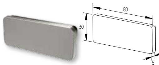
END CAP FOR F50-201 HANDRAIL EMBOUT DE MAIN COURANTE F50-201
