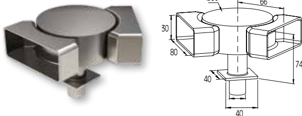
ADJUSTABLE CORNER CONNECTOR FOR 80x30 HANDRAIL WITH F50-102 COLUMN JONCTION ANGULAIRE DE MAIN COURANTE 80x30 AVEC POTEAU F50-102
