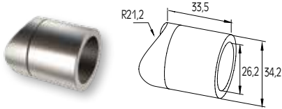
CONNECTOR FOR F50-100 COLUMN WITH PROFILE Ø26 JONCTION DE POTEAU F50-100 AVEC PROFIL Ø26
