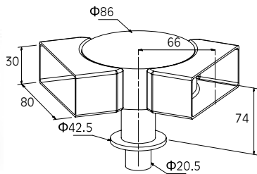
ADJUSTABLE CORNER CONNECTOR FOR HANDRAIL 80x30 WITH COLUMN F50-100 JONCTION ANGULAIRE DE MAIN COURANTE 80x30 AVEC POTEAU F50-100
