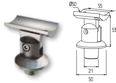
SUPPORT FOR HANDRAIL F50-200 WITH COLUMN F50-101 FIXATION DE MAIN COURANTE F50-200 AVEC POTEAU F50-101
