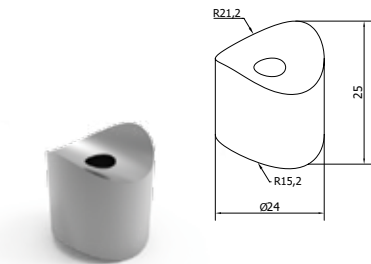
CONNECTOR FOR F50/307-327 WITH F50-103/123 COLUMN JONCTION DE F50-307/327 AVEC POTEAU F50-103/123
