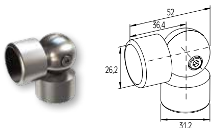
ADJUSTABLE CORNER CONNECTOR FOR PROFILE Ø26 JONCTION ANGULAIRE DE PROFIL Ø26
