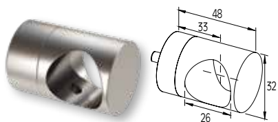
CONNECTOR FOR F50-102 COLUMN WITH PROFILE Ø26 JONCTION DE POTEAU F50-102 AVEC PROFIL Ø26
