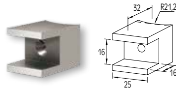
CONNECTOR FOR F50-100 COLUMN WITH F50-302 PROFILE JONCTION DE POTEAU F50-100 AVEC PROFIL F50-302
