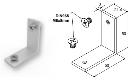
CONNECTOR FOR F50-319 GUIDE EQUERRE DE LIAISON DU GUIDAGE F50-319
