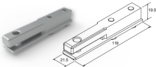
HOLES CALIBRE FOR F50-319 CALIBREUR POUR TROUS DE F50-319
