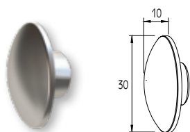
END CAP FOR F50-307 GUIDE EMBOUT DE GUIDAGE F50-307
