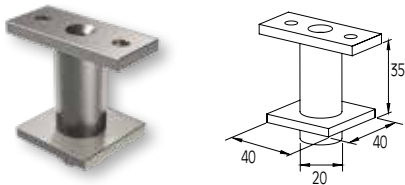
SUPPORT FOR F50-102 COLUMN WITH F50-201 HANDRAIL FIXATION DE POTEAU F50-102 AVEC MAIN COURANTE F50-201
