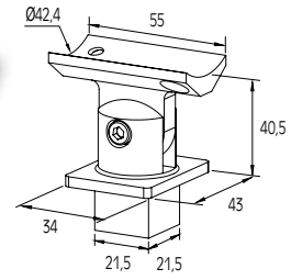
SUPPORT FOR HANDRAIL Ø42 WITH BLADE COLUMN FIXATION DE MAIN COURANTE Ø42 AVEC POTEAU BLADE
