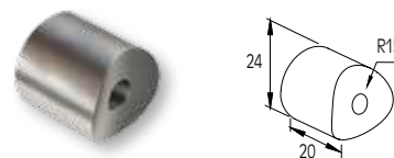
CONNECTOR FOR F50-307 GUIDE WITH F50-102 COLUMN JONCTION DE F50-307 GUIDAGE AVEC POTEAU F50-102
