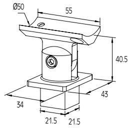
SUPPORT FOR HANDRAIL Ø50 WITH BLADE COLUMN FIXATION DE MAIN COURANTE Ø50 AVEC POTEAU BLADE
