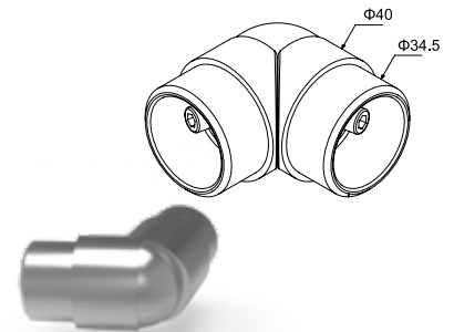
CODE 4371 ADJUSTABLE CORNER CONNECTOR FOR HANDRAIL Ø40 JONCTION ANGULAIRE DE MAIN COURANTE Ø40 PRICE / PRIX 9,55 €/pc
