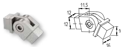
ADJUSTABLE CORNER CONNECTOR FOR F50-302 PROFILE JONCTION ANGULAIRE DE PROFIL F50-302
