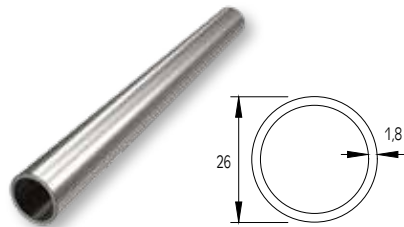
PROFILE Ø26x1.8 PROFILE Ø26x1.8
