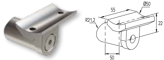
EXTERNAL SUPPORT FOR HANDRAIL Ø50 WITH COLUMN Ø42 FIXATION EXTERIEURE DE MAIN COURANTE Ø50 AVEC POTEAU Ø42
