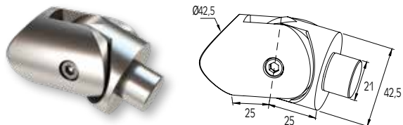
CONNECTOR FOR COLUMN WITH COLUMN F50-100 (STAIRS) JONCTION DE POTEAU AVEC POTEAU F50-100 (ESCALIER)
