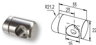
CONNECTOR FOR F50-100 COLUMN WITH PROFILE Ø16 JONCTION DE POTEAU F50-100 AVEC PROFIL Ø16
