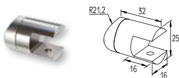
CONNECTOR FOR F50-100 COLUMN WITH F50-302 PROFILE JONCTION DE POTEAU F50-100 AVEC PROFIL F50-302
