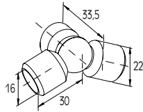
ADJUSTABLE CORNER CONNECTOR FOR PROFILE Ø16 WITH F50-102 COLUMN JONCTION DE PROFIL Ø16 AVEC POTEAU F50-102
