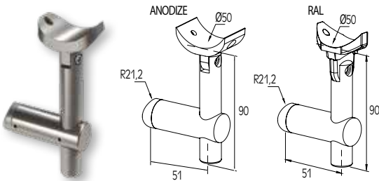
EXTERNAL SUPPORT FOR HANDRAIL Ø50 WITH COLUMN Ø42 FIXATION EXTERIEURE DE MAIN COURANTE Ø50 AVEC POTEAU Ø42
