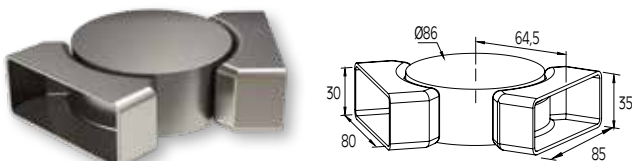
ADJUSTABLE CORNER CONNECTOR FOR F50-201/203 HANDRAIL JONCTION ANGULAIRE DE MAIN COURANTE F50-201/203
