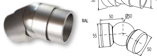
ADJUSTABLE CORNER CONNECTOR FOR COLUMN Ø50 JONCTION ANGULAIRE DE MAIN COURANTE Ø50
