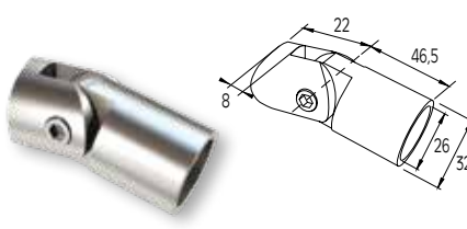
CONNECTOR FOR F50-102 COLUMN WITH PROFILE Ø26 JONCTION DE MAIN COURANTE F50-102 AVEC PROFIL Ø26
