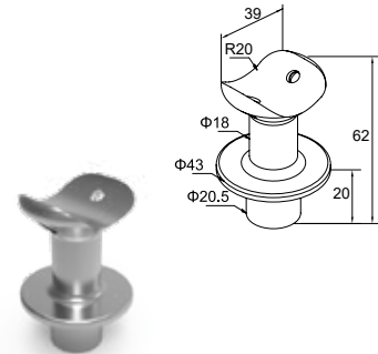
CODE 4368 SUPPORT FOR HANDRAIL Ø40 WITH COLUMN Ø42 FIXATION DE MAIN COURANTE Ø40 AVEC POTEAU Ø42 PRICE / PRIX 3,65 €/pc
