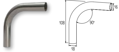
CONNECTOR 90° FOR PROFILE Ø16 JONCTION 90° DE PROFIL Ø16
