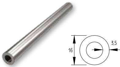
PROFILE Ø16x3.5 PROFIL Ø16x3.5
