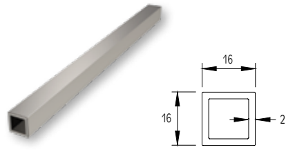
SQUARE 16x16x2 CARE 16x16x2
