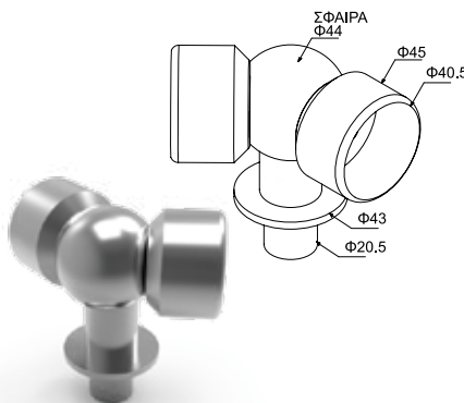
CODE 4370 ADJUSTABLE CORNER CONNECTOR FOR HANDRAIL Ø40 WITH COLUMN Ø42 JONCTION DE MAIN COURANTE Ø40 AVEC POTEAU Ø42 PRICE / PRIX 19,20 €/pc
