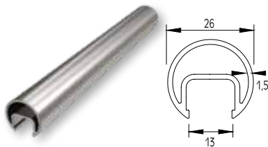
GUIDE FOR GLASS GUIDAGE DE VERRE
