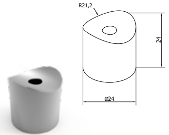
CONNECTOR FOR F50-100 COLUMN WITH F50-102 COLUMN JONCTION DE POTEAU F50-100 AVEC POTEAU F50-102
