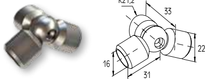
ADJUSTABLE CORNER CONNECTOR FOR PROFILE Ø16 WITH F50-100 COLUMN JONCTION ANGULAIRE DE PROFIL Ø16 AVEC POTEAU F50-100
