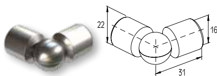
ADJUSTABLE ANGLE CONNECTOR FOR PROFILE Ø16 JONCTION ANGULAIRE DE PROFIL Ø16
