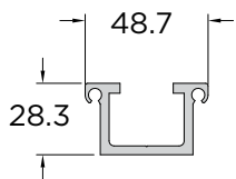
P5302-102 Aluminum Profile (EN AW 6063-T66)
