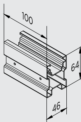
E5310-315 Εξάρτημα σύνδεσης τεγίδων
