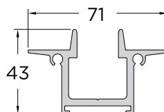
P5302-101 (optional) Aluminum Profile (EN AW 6063-T66)
