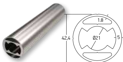
Code/Κωδικός F50-107 Weight/Βάρος 1647 gr/m Length/Μήκος 5.8 m
