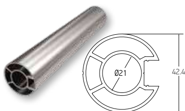
Code/Κωδικός F50-103 Weight/Βάρος 980 gr/m Length/Μήκος 5.8 m
