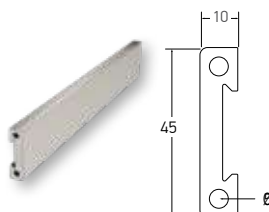
Code/Κωδικός F50-108 Weight/Βάρος 851 gr/m Length/Μήκος 5.8 m
