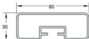
Code/Κωδικός F50-201 Weight/Βάρος 1350 gr/m Length/Μήκος 6 m
