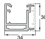
Code/Κωδικός F50-319 Weight/Βάρος 687 gr/m Length/Μήκος 6 m
