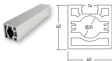
Code/Κωδικός F50-109 Weight/Βάρος 1865 gr/m Length/Μήκος 5.8 m
