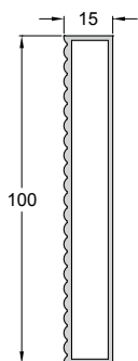
Code/Κωδικός 070-005 IN STOCK Weight/Βάρος 1005 gr/m Length/Μήκος 6 m
