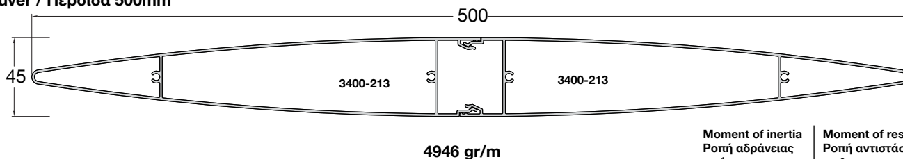
Louver / Περσίδα 500mm
