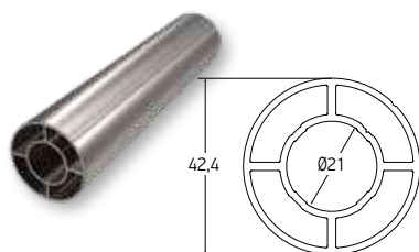
Code/Κωδικός F50-100 Weight/Βάρος 1025 gr/m Length/Μήκος 5.8 m
