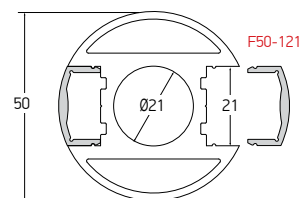
Code/Κωδικός F50-121 Weight/Βάρος 152 gr/m Length/Μήκος 5.8 m
