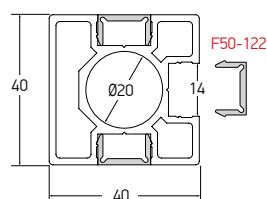
Code/Κωδικός F50-122 Weight/Βάρος 86 gr/m Length/Μήκος 5.8 m
