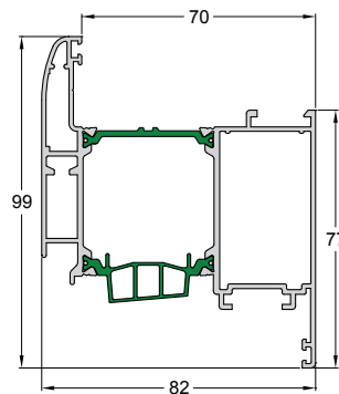
Code/Κωδικός 4750-224 Weight/Βάρος 1973 gr/m Length/Μήκος 6.5 m Pack/Δέμα 2 Bars/Βέργες
