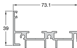
Code/Κωδικός 994-504 Weight/Βάρος 1104 gr/m Length/Μήκος 6 m
