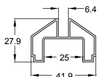
Code/Κωδικός 994-914 Weight/Βάρος 489 gr/m Length/Μήκος 6 m
