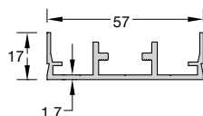
Code/Κωδικός CLS-301 Weight/Βάρος 588 gr/m Length/Μήκος 6 m
