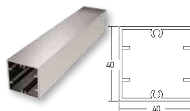
Code/Κωδικός F50-106 Weight/Βάρος 794 gr/m Length/Μήκος 5.8 m
