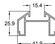
Code/Κωδικός 994-915 Weight/Βάρος 475 gr/m Length/Μήκος 6 m
