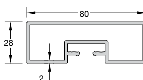
Code/Κωδικός CLS-202 Weight/Βάρος 1360 gr/m Length/Μήκος 6 m
