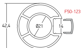
Code/Κωδικός F50-123 Weight/Βάρος 90 gr/m Length/Μήκος 5.8 m
