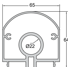
Code/Κωδικός 994-208 Weight/Βάρος 2145 gr/m Length/Μήκος 6 m
