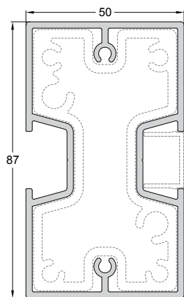
Code/Κωδικός 2200-102 IN STOCK Weight/Βάρος 1885 gr/m Length/Μήκος 6 m
