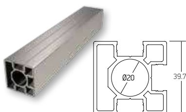
Code/Κωδικός F50-102 Weight/Βάρος 1153 gr/m Length/Μήκος 5.8 m
