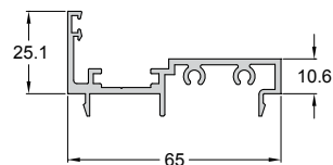
Code/Κωδικός 994-920 Weight/Βάρος 808 gr/m Length/Μήκος 6 m
