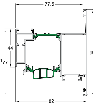
Code/Κωδικός 4750-228 Weight/Βάρος 1922 gr/m Length/Μήκος 6.5 m Pack/Δέμα 2 Bars/Βέργες
