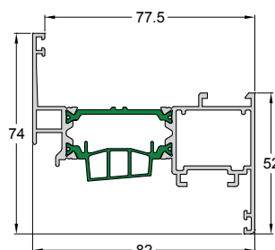
Code/Κωδικός 4750-221 Weight/Βάρος 1418 gr/m Length/Μήκος 6 m Pack/Δέμα 2 Bars/Βέργες
