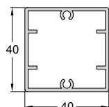
Code/Κωδικός F50-106 Weight/Βάρος 794 gr/m Length/Μήκος 6 m
