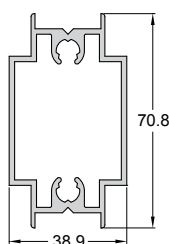
Code/Κωδικός 994-405 Weight/Βάρος 1269 gr/m Length/Μήκος 6 m
