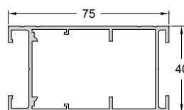
Code/Κωδικός 856 Weight/Βάρος 1115 gr/m Length/Μήκος 6 m
