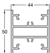
Code/Κωδικός 994-303 Weight/Βάρος 1329 gr/m Length/Μήκος 6 m
