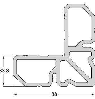
Code/Κωδικός PF31-049 Weight/Βάρος 4713 gr/m Length/Μήκος 6 m Pack/Δέμα 1 Bar/Βέργα
