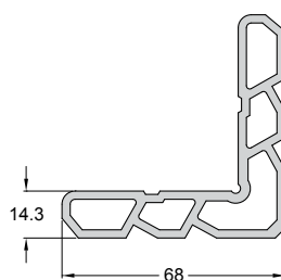
Code/Κωδικός PF31-041 IN STOCK Weight/Βάρος 2022 gr/m Length/Μήκος 6 m Pack/Δέμα 1 Bar/Βέργα
