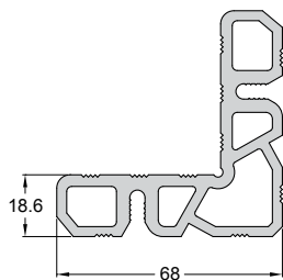
Code/Κωδικός PF31-047 IN STOCK Weight/Βάρος 2772 gr/m Length/Μήκος 6 m Pack/Δέμα 1 Bar/Βέργα
