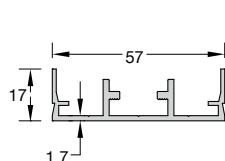
Code/Κωδικός CLS-301 Weight/Βάρος 588 gr/m Length/Μήκος 6 m
