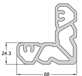
Code/Κωδικός PF31-040 Weight/Βάρος 3241 gr/m Length/Μήκος 6 m Pack/Δέμα 1 Bar/Βέργα
