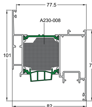
Code/Κωδικός W4750-233 Weight/Βάρος 1882 gr/m Length/Μήκος 6.5 m Pack/Δέμα 2 Bars/Βέργες
