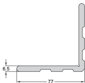
Code/Κωδικός PF31-001 IN STOCK Weight/Βάρος 2225 gr/m Length/Μήκος 6 m Pack/Δέμα 1 Bar/Βέργα
