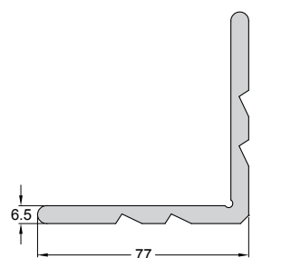
Code/Κωδικός PF31-042 IN STOCK Weight/Βάρος 2364 gr/m Length/Μήκος 6 m Pack/Δέμα 1 Bar/Βέργα
