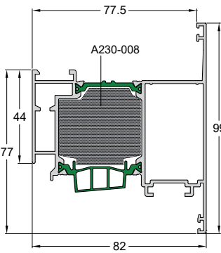
Code/Κωδικός W4750-228 Weight/Βάρος 1922 gr/m Length/Μήκος 6.5 m Pack/Δέμα 2 Bars/Βέργες
