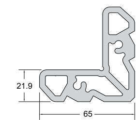
Code/Κωδικός PF031-084 Weight/Βάρος 3472 gr/m Length/Μήκος 6 m Pack/Δέμα 1 Bar/Βέργα
