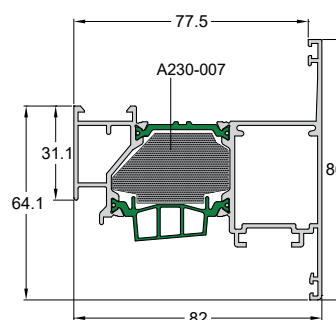
Code/Κωδικός W4750-227 Weight/Βάρος 1704 gr/m Length/Μήκος 6 m Pack/Δέμα 2 Bars/Βέργες
