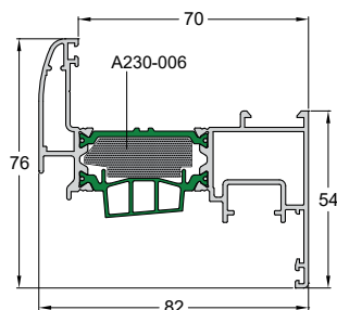
Code/Κωδικός W4750-235 Weight/Βάρος 1946 gr/m Length/Μήκος 6.5 m Pack/Δέμα 2 Bars/Βέργες
