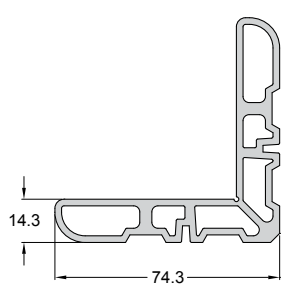
Code/Κωδικός PF31-010 IN STOCK Weight/Βάρος 2209 gr/m Length/Μήκος 6 m Pack/Δέμα 1 Bar/Βέργα
