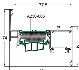
Code/Κωδικός W4750-221 Weight/Βάρος 1418 gr/m Length/Μήκος 6 m Pack/Δέμα 2 Bars/Βέργες
