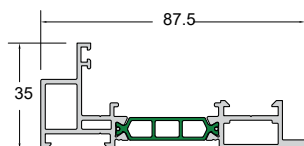
Code/Κωδικός W85-105 Weight/Βάρος 1076 gr/m Length/Μήκος 6 m Pack/Δέμα 2 Bars/Βέργες
