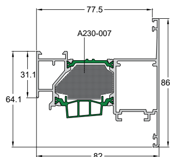
Code/Κωδικός W4750-227 Weight/Βάρος 1704 gr/m Length/Μήκος 6 m Pack/Δέμα 2 Bars/Βέργες
