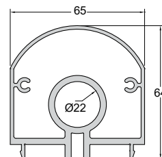
Code/Κωδικός P994-208 Weight/Βάρος 2145 gr/m Length/Μήκος 6 m
