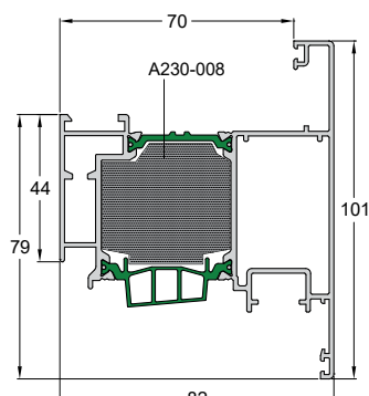
Code/Κωδικός W4750-218 Weight/Βάρος 1988 gr/m Length/Μήκος 6.5 m Pack/Δέμα 2 Bars/Βέργες
