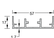
Code/Κωδικός CLS-301 Weight/Βάρος 588 gr/m Length/Μήκος 6 m
