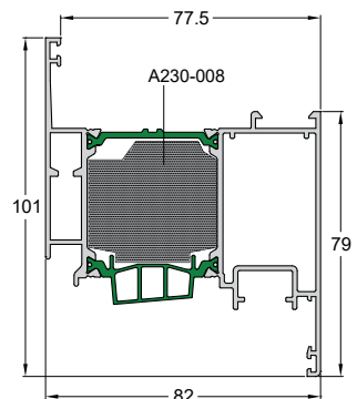
Code/Κωδικός W4750-233 Weight/Βάρος 1882 gr/m Length/Μήκος 6.5 m Pack/Δέμα 2 Bars/Βέργες
