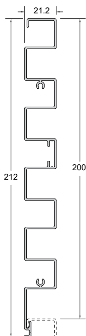
Code/Κωδικός WD-2020 Weight/Βάρος 1479 gr/m Length/Μήκος 6 m Pack/Δέμα 2 Bars/Βέργες
