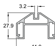
Code/Κωδικός P992-904 Weight/Βάρος 651 gr/m Length/Μήκος 6 m
