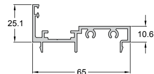
Code/Κωδικός P994-920 Weight/Βάρος 808 gr/m Length/Μήκος 6 m
