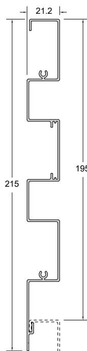
Code/Κωδικός WD-2040 Weight/Βάρος 1236 gr/m Length/Μήκος 6 m Pack/Δέμα 2 Bars/Βέργες
