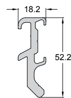
Code/Κωδικός PF31-034 IN STOCK Weight/Βάρος 940 gr/m Length/Μήκος 6 m Pack/Δέμα 1 Bar/Βέργα
