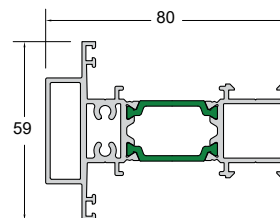
Code/Κωδικός W85-303 Weight/Βάρος 1728 gr/m Length/Μήκος 6 m Pack/Δέμα 2 Bars/Βέργες
