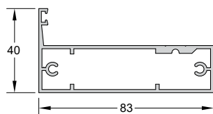
Code/Κωδικός GF75-101 Weight/Βάρος 1166 gr/m Length/Μήκος 6 m Pack/Δέμα 3 Bars/Βέργες
