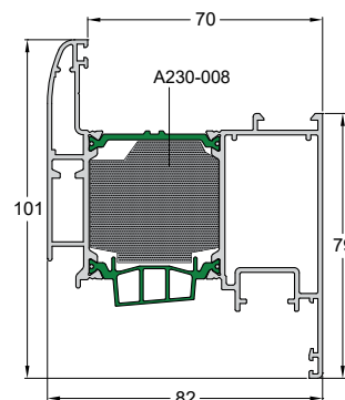
Code/Κωδικός W4750-234 Weight/Βάρος 1989 gr/m Length/Μήκος 6.5 m Pack/Δέμα 2 Bars/Βέργες
