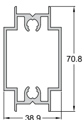
Code/Κωδικός P994-405 Weight/Βάρος 1269 gr/m Length/Μήκος 6 m
