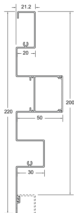
Code/Κωδικός WD-2050 Weight/Βάρος 1523 gr/m Length/Μήκος 6 m Pack/Δέμα 2 Bars/Βέργες
