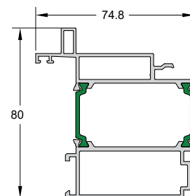
Code/Κωδικός W85-911 Weight/Βάρος 1823 gr/m Length/Μήκος 6 m Pack/Δέμα 2 Bars/Βέργες
