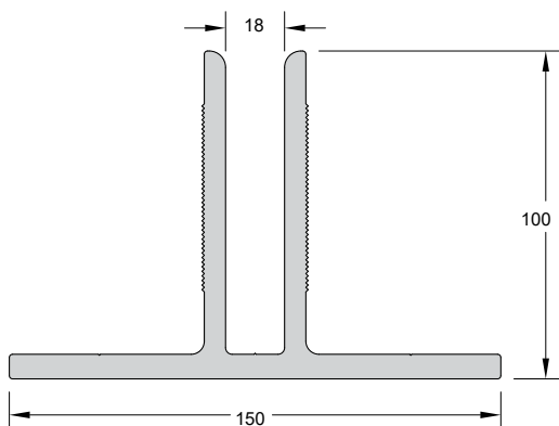
Code/Κωδικός CW35-909 Weight/Βάρος 6383 gr/m Length/Μήκος 6 m Pack/Δέμα 1 Bar/Βέργα
