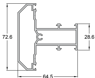
Code/Κωδικός P994-301 Weight/Βάρος 1484 gr/m Length/Μήκος 6 m
