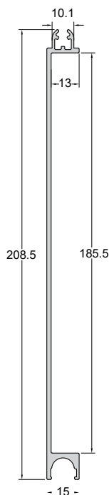
Code/Κωδικός P994-922 Weight/Βάρος 1384 gr/m Length/Μήκος 6 m
