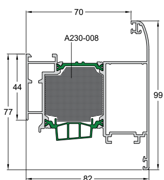
Code/Κωδικός W4750-226 Weight/Βάρος 1962 gr/m Length/Μήκος 6.5 m Pack/Δέμα 2 Bars/Βέργες
