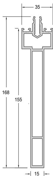
Code/Κωδικός CW35-506 Weight/Βάρος 2370 gr/m Length/Μήκος 6.5 m Pack/Δέμα 2 Bars/Βέργες
