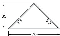
Code/Κωδικός SH3200-627 Weight/Βάρος 703 gr/m Length/Μήκος 6 m Pack/Δέμα 4 Bars/Βέργες
