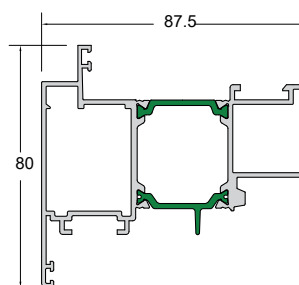
Code/Κωδικός W85-205 Weight/Βάρος 1896 gr/m Length/Μήκος 6 m Pack/Δέμα 2 Bars/Βέργες
