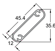
Code/Κωδικός SH3200-623 Weight/Βάρος 430 gr/m Length/Μήκος 6 m Pack/Δέμα 6 Bars/Βέργες
