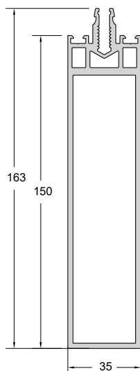
Code/Κωδικός CW35-502 Weight/Βάρος 3048 gr/m Length/Μήκος 6.5 m Pack/Δέμα 1 Bars/Βέργες
