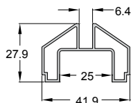
Code/Κωδικός P994-914 Weight/Βάρος 489 gr/m Length/Μήκος 6 m
