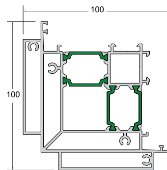
Code/Κωδικός W85-903 Weight/Βάρος 3746 gr/m Length/Μήκος 6 m Pack/Δέμα 1 Bars/Βέργες
