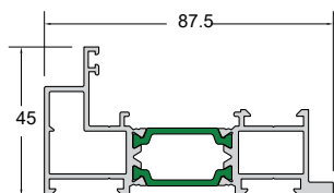
Code/Κωδικός W85-104 Weight/Βάρος 1448 gr/m Length/Μήκος 6 m Pack/Δέμα 2 Bars/Βέργες
