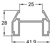
Code/Κωδικός P992-903 Weight/Βάρος 532 gr/m Length/Μήκος 6 m
