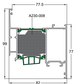
Code/Κωδικός W4750-223 Weight/Βάρος 1866 gr/m Length/Μήκος 6.5 m Pack/Δέμα 2 Bars/Βέργες
