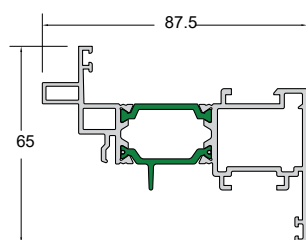
Code/Κωδικός W85-203 Weight/Βάρος 1550 gr/m Length/Μήκος 6 m Pack/Δέμα 2 Bars/Βέργες
