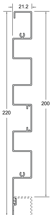
Code/Κωδικός WD-2030 Weight/Βάρος 1382 gr/m Length/Μήκος 6 m Pack/Δέμα 2 Bars/Βέργες
