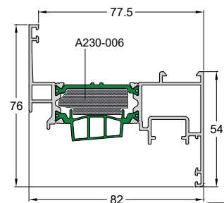
Code/Κωδικός W4750-231 Weight/Βάρος 1421 gr/m Length/Μήκος 6 m Pack/Δέμα 2 Bars/Βέργες
