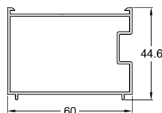
Code/Κωδικός SH3200-907 Weight/Βάρος 767 gr/m Length/Μήκος 6 m Pack/Δέμα 2 Bars/Βέργες
