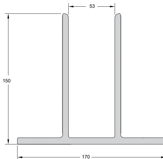
Code/Κωδικός EW50-943 Weight/Βάρος 8691 gr/m Length/Μήκος 6 m Pack/Δέμα 1 Bar/Βέργα
