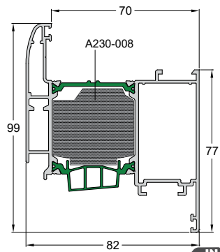
Code/Κωδικός W4750-224 Weight/Βάρος 1973 gr/m Length/Μήκος 6.5 m Pack/Δέμα 2 Bars/Βέργες
