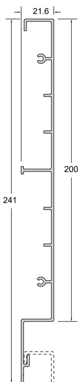
Code/Κωδικός WD-2001 Weight/Βάρος 1597 gr/m Length/Μήκος 6 m Pack/Δέμα 2 Bars/Βέργες
