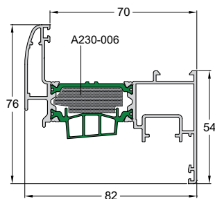
Code/Κωδικός W4750-235 Weight/Βάρος 1946 gr/m Length/Μήκος 6.5 m Pack/Δέμα 2 Bars/Βέργες
