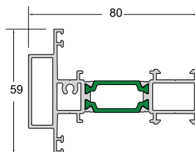
Code/Κωδικός W85-302 Weight/Βάρος 1584 gr/m Length/Μήκος 6 m Pack/Δέμα 2 Bars/Βέργες
