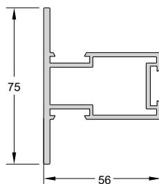
Code/Κωδικός GF75-201 Weight/Βάρος 1472 gr/m Length/Μήκος 6 m Pack/Δέμα 2 Bars/Βέργες
