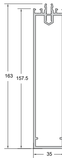
Code/Κωδικός CW35-504 Weight/Βάρος 2824 gr/m Length/Μήκος 6.5 m Pack/Δέμα 2 Bars/Βέργες
