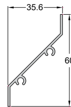
Code/Κωδικός SH3200-621 Weight/Βάρος 358 gr/m Length/Μήκος 6 m Pack/Δέμα 2 Bars/Βέργες
