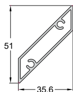
Code/Κωδικός SH3200-622 Weight/Βάρος 525 gr/m Length/Μήκος 6 m Pack/Δέμα 5 Bars/Βέργες
