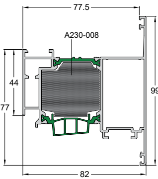
Code/Κωδικός W4750-228 Weight/Βάρος 1922 gr/m Length/Μήκος 6.5 m Pack/Δέμα 2 Bars/Βέργες
