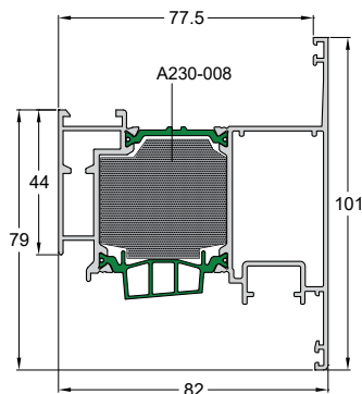
Code/Κωδικός W4750-235 Weight/Βάρος 1946 gr/m Length/Μήκος 6.5 m Pack/Δέμα 2 Bars/Βέργες
