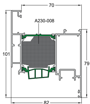
Code/Κωδικός W4750-217 Weight/Βάρος 1926 gr/m Length/Μήκος 6.5 m Pack/Δέμα 2 Bars/Βέργες
