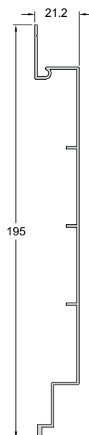
Code/Κωδικός P070-015 Weight/Βάρος 850 gr/m Length/Μήκος 6 m Pack/Δέμα 2 Bars/Βέργες
