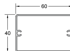
Code/Κωδικός SH3200-628 Weight/Βάρος 742 gr/m Length/Μήκος 6 m Pack/Δέμα 2 Bars/Βέργες
