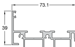
Code/Κωδικός P994-504 Weight/Βάρος 1104 gr/m Length/Μήκος 6 m
