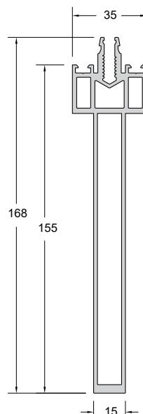
Code/Κωδικός CW35-505 Weight/Βάρος 2486 gr/m Length/Μήκος 6.5 m Pack/Δέμα 2 Bars/Βέργες
