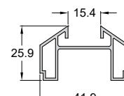
Code/Κωδικός P994-915 Weight/Βάρος 475 gr/m Length/Μήκος 6 m
