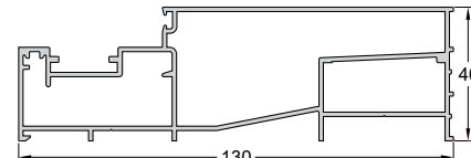
Code/Κωδικός SH3200-105 Weight/Βάρος 1660 gr/m Length/Μήκος 6 m Pack/Δέμα 2 Bars/Βέργες
