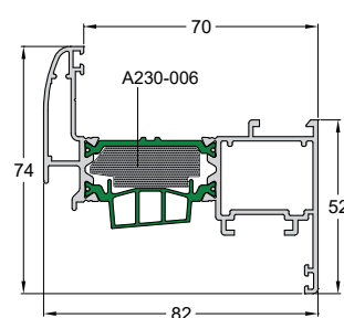
Code/Κωδικός W4750-228 Weight/Βάρος 1922 gr/m Length/Μήκος 6.5 m Pack/Δέμα 2 Bars/Βέργες
