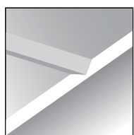
Χάραξη σχήματος V μέγιστο βάθος 0.8mm V-shape engraving maximum depth 0.8mm
