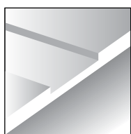
Χάραξη σχήματος U βάθος 0.8mm - πλάτος 10/20mm U-shape engraving depth 0.8mm - width 10/20mm
