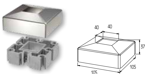
ΠΕΛΜΑ ΣΤΗΡΙΞΗΣ ΓΙΑ ΚΟΛΩΝΑ 40x40 SUPPORT FOOT FOR 40x40 COLUMN
