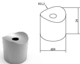
ΣΥΝΔΕΣΜΟΣ ΚΟΛΩΝΑΣ F50-100 ΜΕ ΚΟΛΩΝΑ F50-102 CONNECTOR FOR F50-100 COLUMN WITH F50-102 COLUMN
