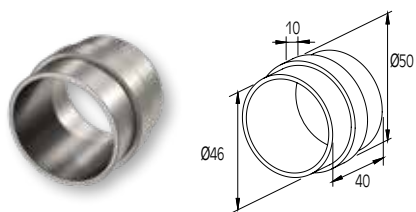
ΕΣΩΤΕΡΙΚΟΣ ΣΥΝΔΕΣΜΩΝ ΚΟΥΡΑΣΤΩΝ Ø50 CONNECTOR FOR HANDRAIL Ø50 (INTERNAL)
