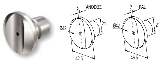
ΣΥΝΔΕΣΜΟΣ ΚΟΛΩΝΑΣ ΜΕ ΚΟΛΩΝΑ F50-100 CONNECTOR FOR COLUMN WITH COLUMN F50-100
