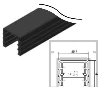
EPDM GASKET Code F85-464 for glass / pour verre 17.52 & 16.76 mm
