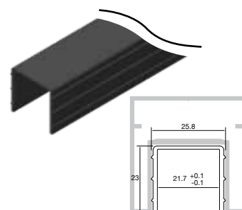
EPDM GASKET Code F85-465 for glass / pour verre 21.52 mm
