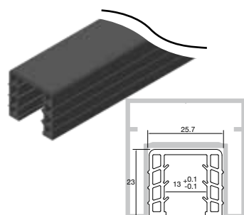
EPDM GASKET Code F85-463 for glass / pour verre 13.52 & 12.76 mm
