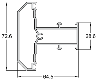
Code/Κωδικός 994-301 Weight/Βάρος 1484 gr/m Length/Μήκος 6 m
