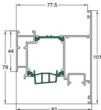
Code/Κωδικός 4750-235 Weight/Βάρος 1946 gr/m Length/Μήκος 6.5 m Pack/Δέμα 2 Bars/Βέργες
