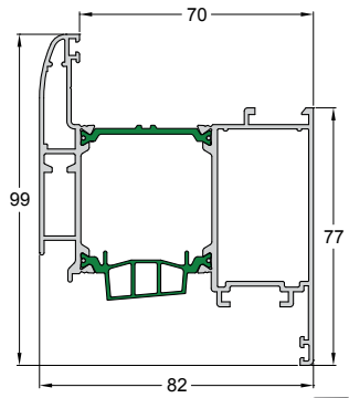
Code/Κωδικός 4750-224 IN STOCK Weight/Βάρος 1973 gr/m Length/Μήκος 6.5 m Pack/Δέμα 2 Bars/Βέργες
