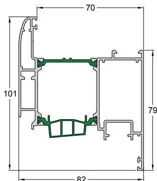
Code/Κωδικός 4750-234 Weight/Βάρος 1989 gr/m Length/Μήκος 6.5 m Pack/Δέμα 2 Bars/Βέργες
