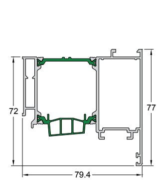
Code/Κωδικός 4750-229 Weight/Βάρος 1694 gr/m Length/Μήκος 6.5 m Pack/Δέμα 2 Bars/Βέργες
