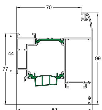
Code/Κωδικός 4750-226 Weight/Βάρος 1962 gr/m Length/Μήκος 6.5 m Pack/Δέμα 2 Bars/Βέργες
