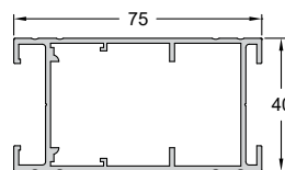
Code/Κωδικός 856 Weight/Βάρος 1115 gr/m Length/Μήκος 6 m
