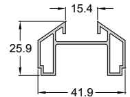
Code/Κωδικός 994-915 Weight/Βάρος 475 gr/m Length/Μήκος 6 m
