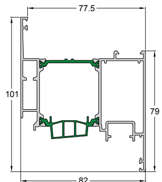
Code/Κωδικός 4750-233 Weight/Βάρος 1882 gr/m Length/Μήκος 6.5 m Pack/Δέμα 2 Bars/Βέργες
