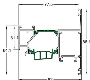
Code/Κωδικός 4750-227 Weight/Βάρος 1704 gr/m Length/Μήκος 6 m Pack/Δέμα 2 Bars/Βέργες
