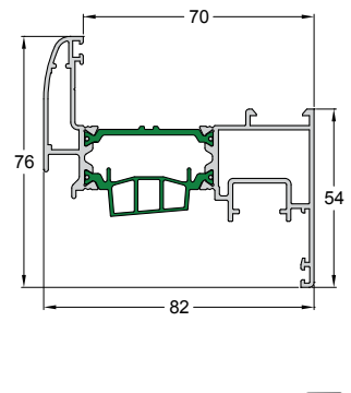
Code/Κωδικός 4750-232 IN STOCK Weight/Βάρος 1496 gr/m Length/Μήκος 6 m Pack/Δέμα 2 Bars/Βέργες
