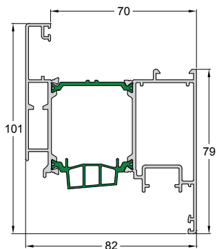
Code/Κωδικός 4750-217 Weight/Βάρος 1926 gr/m Length/Μήκος 6.5 m Pack/Δέμα 2 Bars/Βέργες
