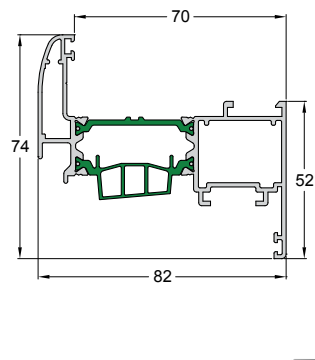
Code/Κωδικός 4750-222 IN STOCK Weight/Βάρος 1493 gr/m Length/Μήκος 6 m Pack/Δέμα 2 Bars/Βέργες
