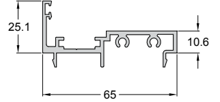
Code/Κωδικός 994-920 Weight/Βάρος 808 gr/m Length/Μήκος 6 m
