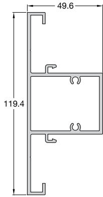
Code/Κωδικός 994-302 Weight/Βάρος 1815 gr/m Length/Μήκος 6 m
