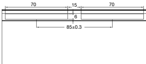
ΔΙΑΤΡΗΣΗ / PERFORATION
