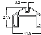
Code/Κωδικός 992-904 Weight/Βάρος 651 gr/m Length/Μήκος 6 m
