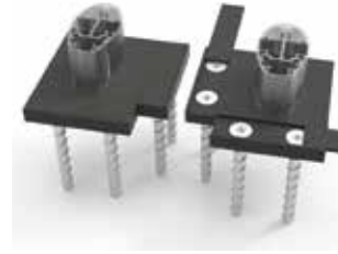
Κωδικός / Code: 4736 ΓΩΝΙΑΚΟ ΠΕΛΜΑ ΚΟΛΩΝΑΣ FSN-102 CORNER SUPPORT FOOT FOR COLUMN FSN-102
