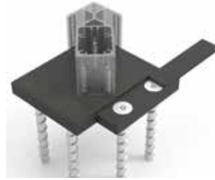
Κωδικός / Code: 4735 ΠΕΛΜΑ ΚΟΛΩΝΑΣ FSN-104 SUPPORT FOOT FOR COLUMN FSN-104
